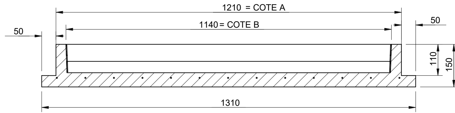
Section D-D
